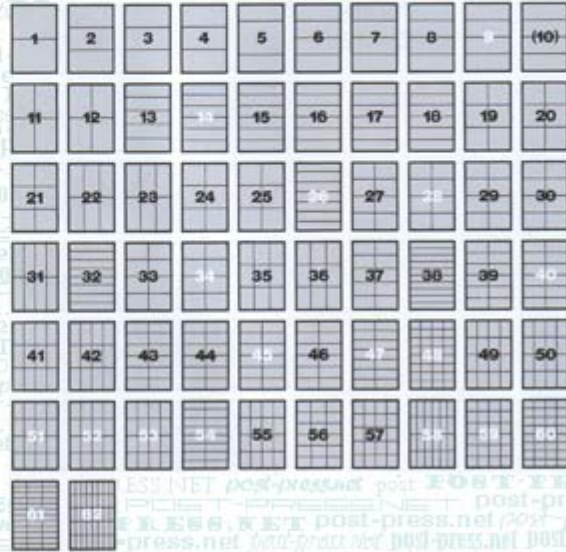
Возможные виды фальцев на фальцовке MBO K66-4S KTL
